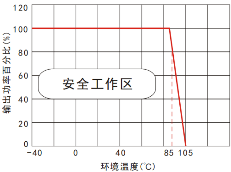
温度降额曲线图
