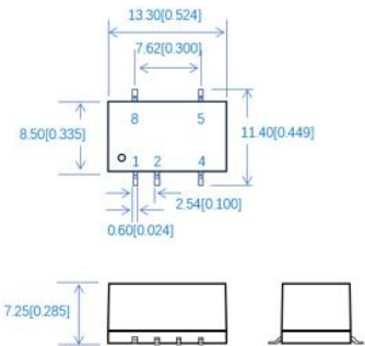
图4：外型尺寸
