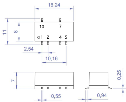
图4：外型尺寸
