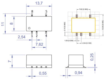
图4：外型尺寸
