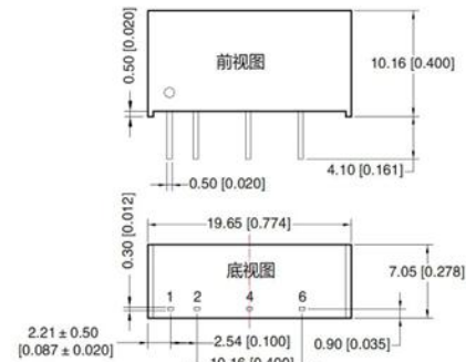
图4：外型尺寸
