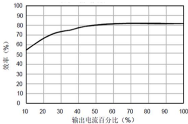
图2：效率VS输出负载（标称电压输入）
