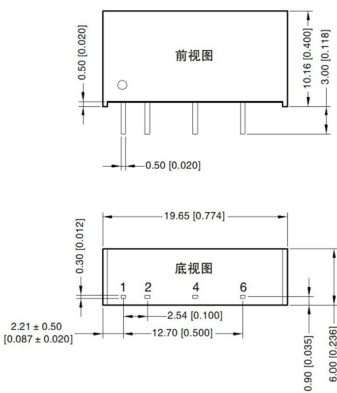
图3：外型尺寸
