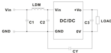
图5：EMC 典型推荐电路
