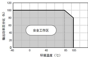
图1：温度降额曲线图
