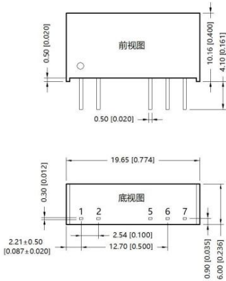
图4：外型尺寸
