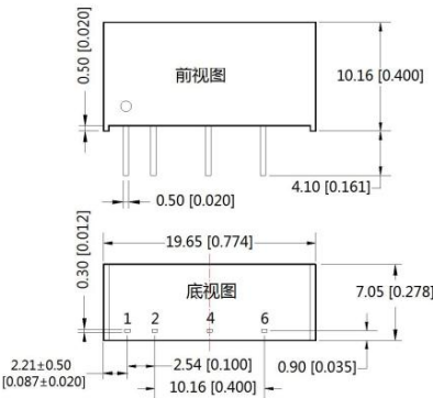
图3：外型尺寸
