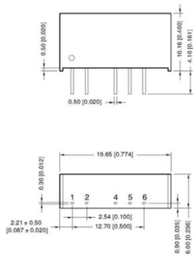
图4：外型尺寸
