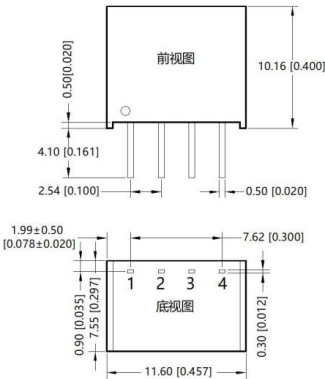
图4：外型尺寸
