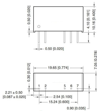
图4：外型尺寸
