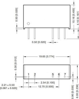
图4：外型尺寸
