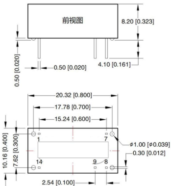
图4：外型尺寸
