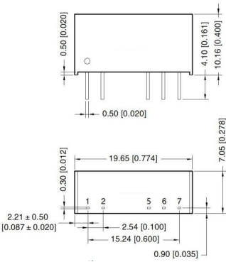
图4：外型尺寸
